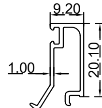
كليس دفة زجاج 9 ملم الرقم التسلسلي للصنف: BLT4395 الوزن 0.183:(Kg/m)
