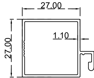
منخل (27 / 27) ملم الرقم التسلسلي للصنف: BLT361 الوزن 0.365:(Kg/m)
