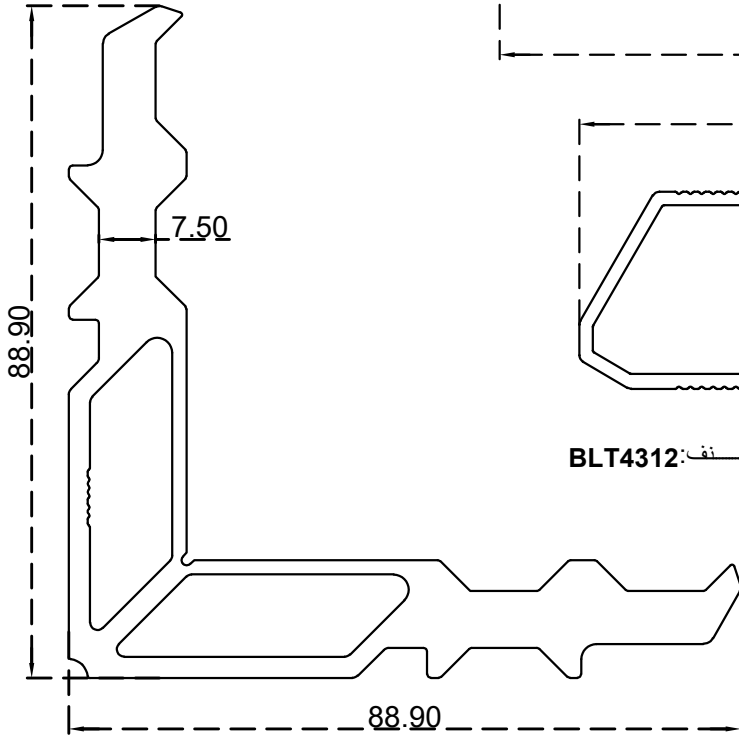
زاوية جمع حلق 2200 الرقم التسلسلي للصنف: BLT4631 الوزن 3.335:(Kg/m)
