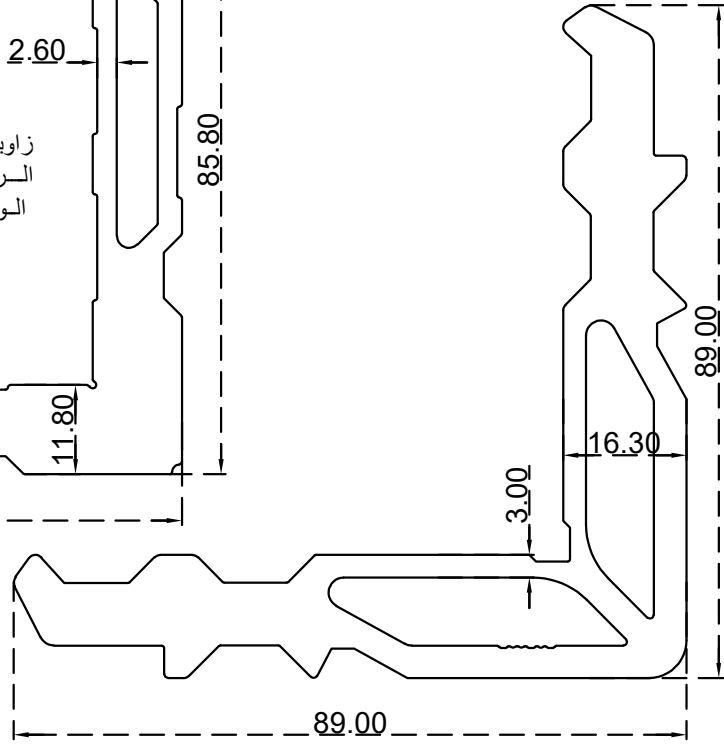
زاوية جمع حلق 2200 الرقم التسلسلي للصنف: BLT4321 الوزن 4.058:(Kg/m)
