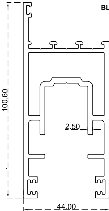
دفة 100 ملم الرقم التسلسلي للصنف: BLT4384 الوزن 2.306:(Kg/m)
