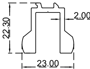
يو علوي الرقم التسلسلي للصنف: BLT4392 الوزن 0.475:(Kg/m)
