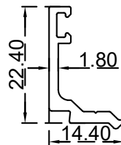
كليس دفة زجاج 4 ملم الرقم التسلسلي للصنف: BLT4394 الوزن 0.196:(Kg/m)
