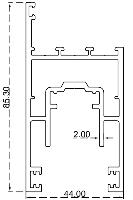
دفة 85 ملم الرقم التسلسلي للصنف: BLT4383 الوزن 1.862:(Kg/m)
