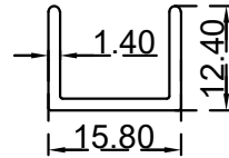
مقوي امباطية الرقم التسلسلي للصنف: BLT4391 الوزن 0.143:(Kg/m)
