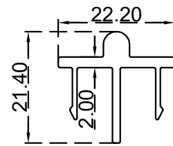
غطاء مجرى الرقم التسلسلي للصنف: BLT4390 الوزن 0.290:(Kg/m)
